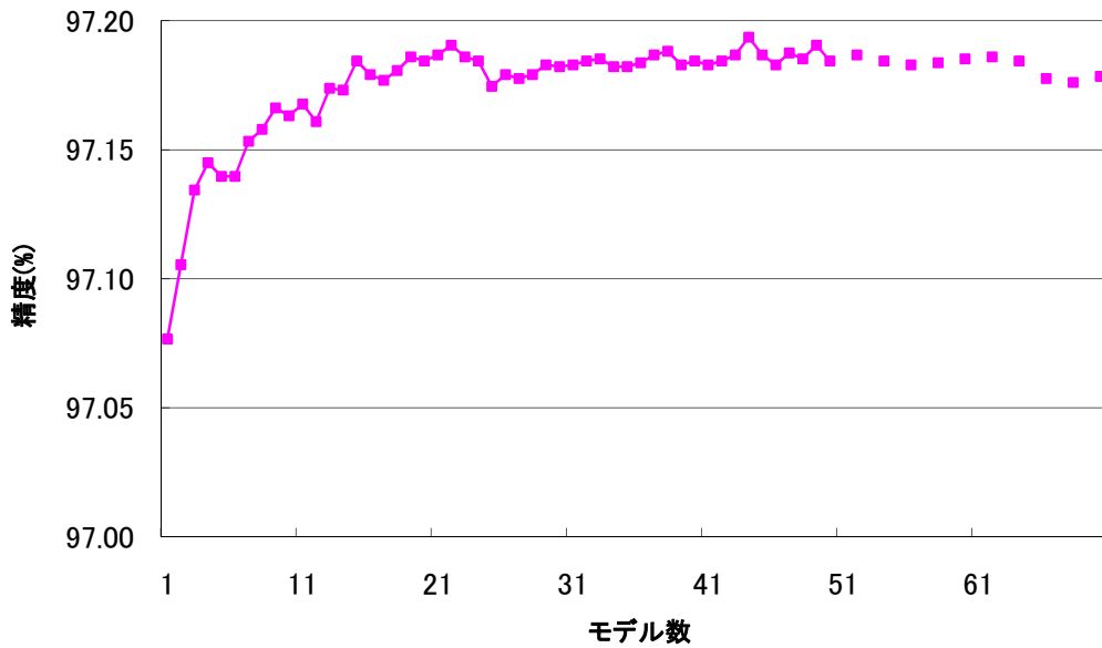
図 2: BPM におけるモデルの数に対する精度
