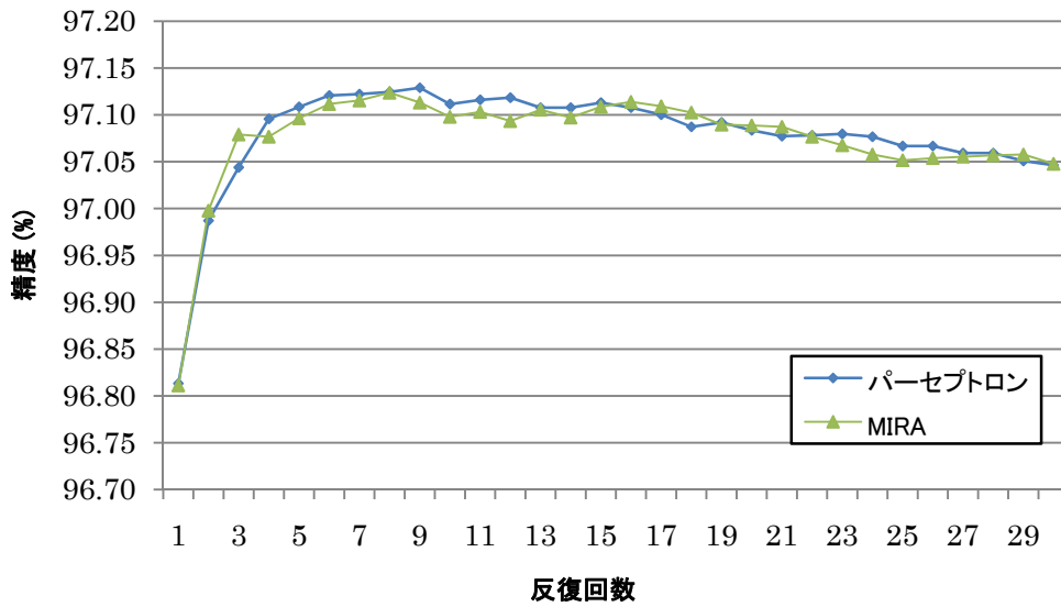
図 1: パーセプトロンと MIRA に対する反復回数と精度の関係
