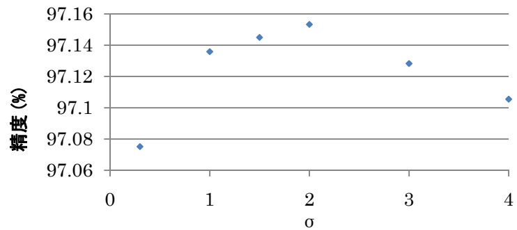
図 3: CRF の development データに対する \sigma と精度の関係
